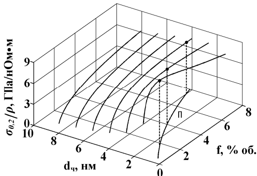
Рис. 2 – Зависимость параметра оптимизации от f и d_c : ● – локальный максимум параметра оптимизации, линия П – проекция локальных максимумов на плоскость d_c - f .
