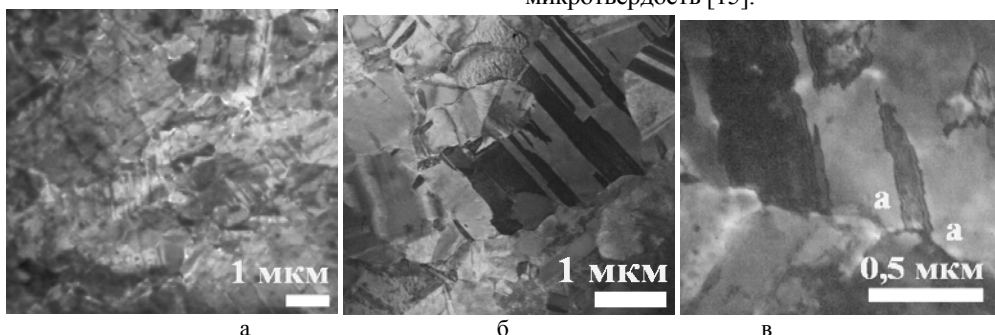
Рис. 6 – Влияние отжига 600^\circ\text{C} (2 часа) на структуру низкотемпературных пленок меди: а – исходное состояние, б, в – поле отжига.
