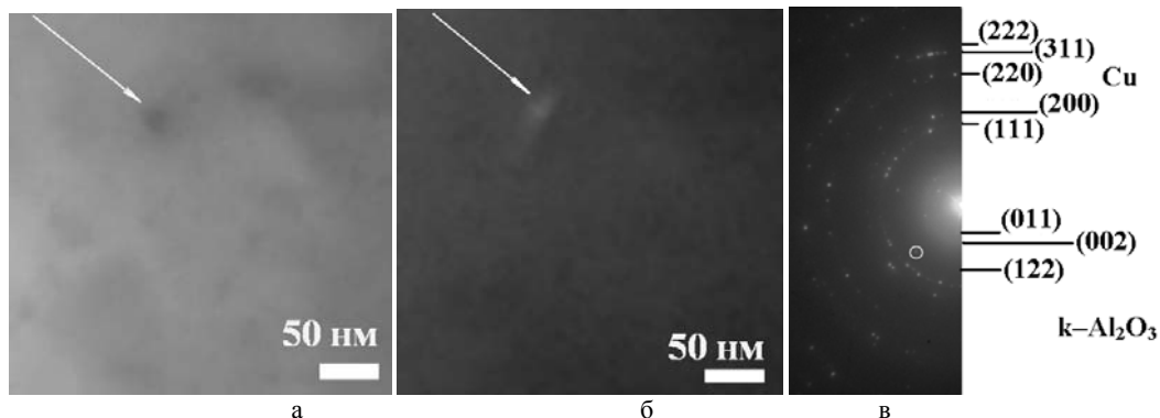
Рис. 3 – Электронно-микроскопическое изображение частиц Al_2O_3 в исходном состоянии композита ( T_n > 300 °С), электролитически утоненные образцы: а – светлое поле; б – темное поле; в – дифракция
