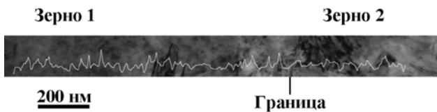
Рис. 5 – EDS сигнал Al привязанный к микроструктуре
