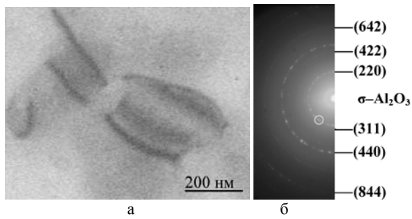
Рис. 4 – Электронно-микроскопическое изображение крупных частиц \text{Al}_2\text{O}_3 после отжига композита ( T_n > 300^\circ\text{C} ), углеродная экстракционная реплика: а – светлое поле; б – дифракция
