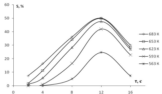
Рис. 2 – Вплив зміни часу контакту на селективність утворення цільових продуктів ММА і МАК, в інтервалі температур 563–683 К.
