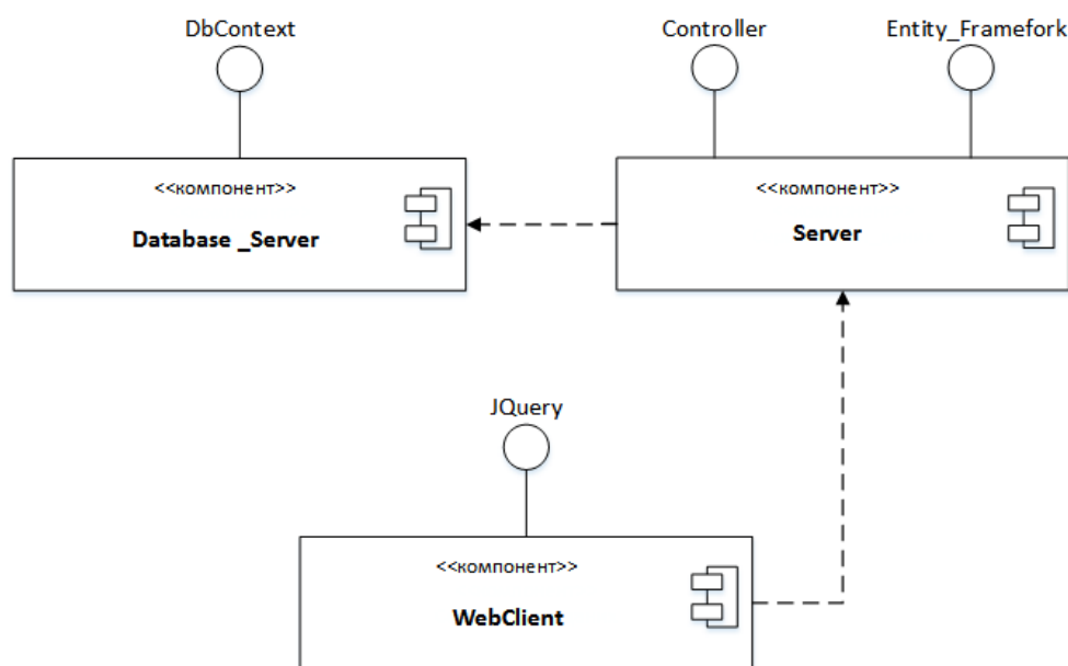
Рис. 1 – Діаграма компонентів
