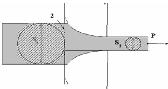
Рис. 1 – Схематическое изображение процесса волочения: 1 – фильера (волока), 2 – заготовка (пруток), S_1 и S_2 – площадь поперечного сечения прутка до и после волочения, \rightarrow – направление приложения усилия P для волочения.
