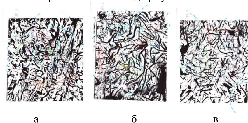
Рис. 2 – Мікроструктури чавуну, модифікованого феросиліцієм ФС65Ба4, x100 а – початковий момент модифікування, б – через 10 хв. після модифікування, в – через 15 хв. після модифікування
