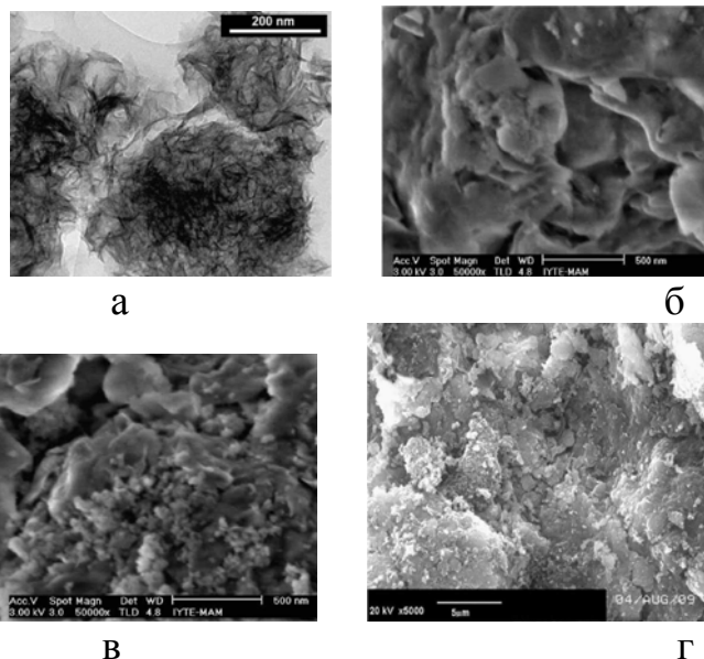
Рис. 3 – Електронномікроскопічні знімки зразків Zn- стивенситу: а – Zn-СТ; б – AlPILC; в – CrPILC; г – TiPILC
