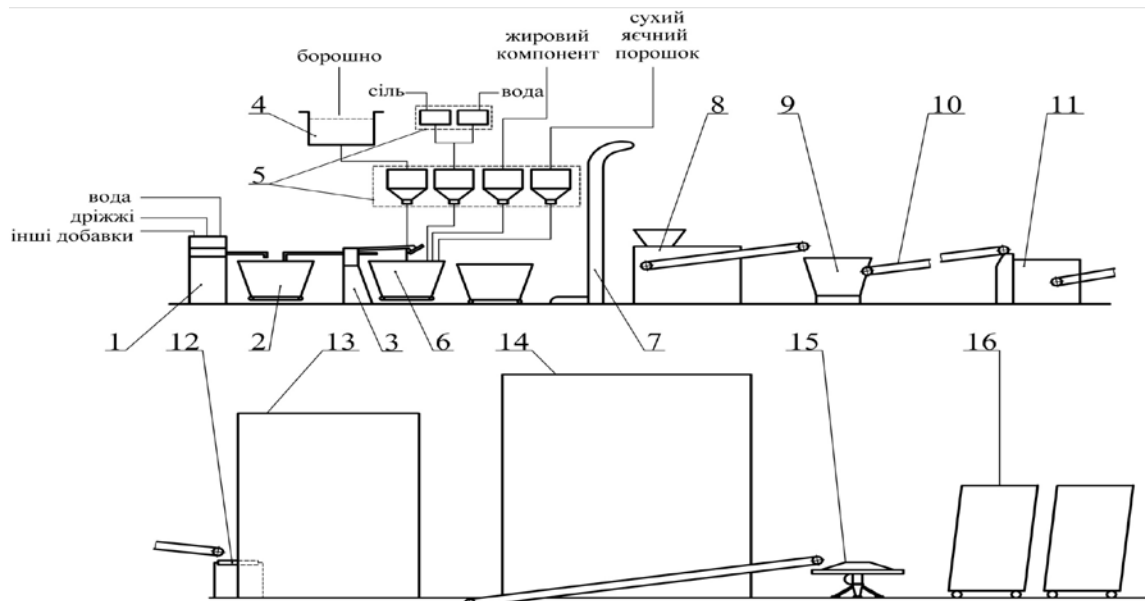
Рис. 2 – Апаратурна схема технологічного процесу виробництва дріжджових виробів з використання СКД: 1 – дозувальна станція; 2 – конвекційна діжка для активації дріжджів; 3 – тістомісильна машина; 4 – просіювач борошна; 5 – дозатори; 6 – діжка; 7 – діжоопрокидувач; 8 – тісторозділювач; 9 – округлювач; 10 – транспортер; 11* – закатувальна машина; 12* – укладач; 13 – розстоювальна шафа; 14 – пароконвекційна піч; 15 – циркуляційний стіл; 16 – контейнер; *- апаратурне устаткування, що використовують для отримання подових виробів
